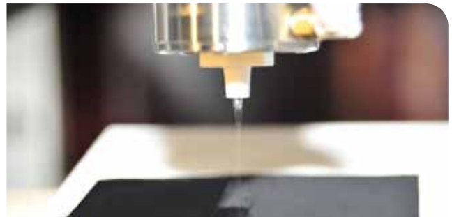
Direkte Membranabscheidung auf die Elektrodenstrukturen mittels Ultraschall-Spray-Beschichtung
