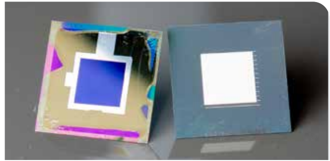
Die Perowskit-Silizium-Tandemsolarzelle beruht auf zwei Innovationen: einer nanotexturierten Frontseite (links) und einer Rückseite mit dielektrischem Reflektor (rechts).
