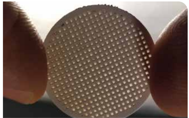
Membranträger aus Magnesiumoxid (MgO), der mittels 3D-Siebdruck hergestellt wurde
